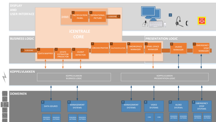
Figuur 1 Structuurschema
